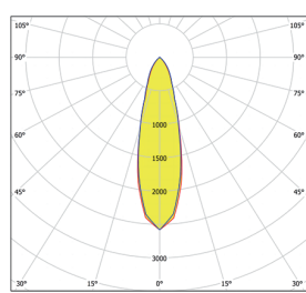
AN10D7H30G 30°
