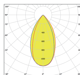
AN10D7H60G 60°
