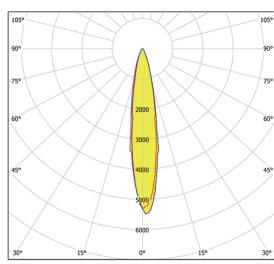
AN10D7H15G 15°
