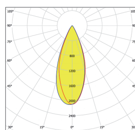
AN10D7H40G 40°
