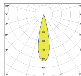
AN10D7H25G 25°
