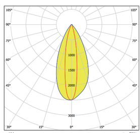
AN10D7H1560G 15x60°
